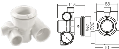
32 Mm Hava ve 50 Su ıkıřlı 32 Mm Air and 50 Water Outlet
