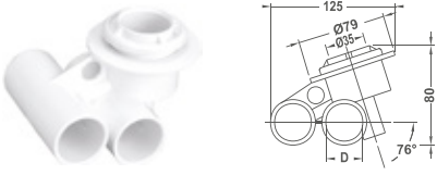
32 Mm Hava ve 32 Su ıkıřlı 32 Mm Air and 32 Water Outlet
